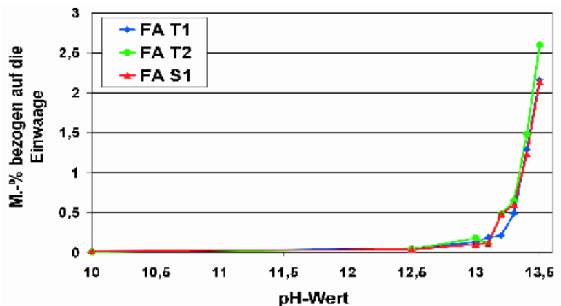
Bild 3: Die gelösten Anteile \text{SiO}_2 dreier Steinkohlenflugaschen nach einem Monat Lagerung in \text{NaOH} in Abhängigkeit vom pH-Wert (T = Trockenfeuerung, S = Schmelzkammerfeuerung)
