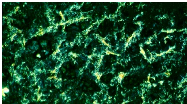
Bild 1: Polarisationsmikroskopische Aufnahme des dreidimensional vernetzten \text{Ca}(\text{OH})_2 -Gefüges (aus [5]) (hell: \text{Ca}(\text{OH})_2 dunkel: CSH-Phasen oder Klinkerkörner)
