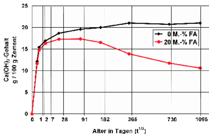
Bild 2: Die Abnahme des \text{Ca}(\text{OH})_2 -Gehalts mit der Zeit bei Einsatz von Steinkohlenflugasche in Portlandzementbeton ( w/(z+f) = 0,6 ) (aus [3])
